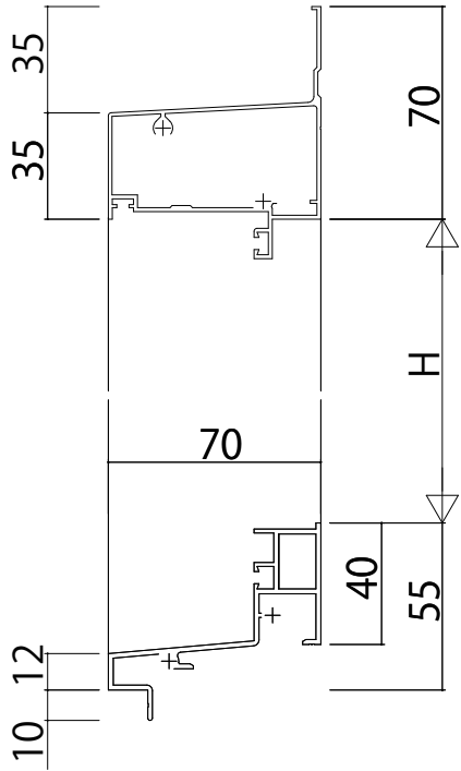
(84) ドア【フラッシュタイプ・通風ドア】 鉄骨枠 外付
