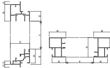
(6) 引違い窓・片引き窓・両軸片引き窓・引分け窓・自由片引き窓 自立(つらいち枠) アンクルなし
