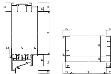
(10) 引違い窓・片引き窓(下枠フラット仕様) RC枠 アンクル付
