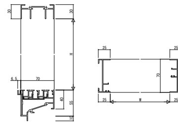
(11) 引違い窓・片引き窓(下枠フラット仕様) RC枠 アンクルなし
