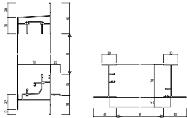
(8) 引違い窓・片引き窓・両軸片引き窓・引分け窓・自由片引き窓 鉄骨枠 外付
