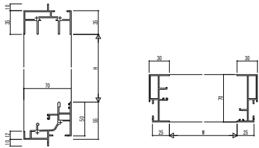
(5) 引違い窓・片引き窓・両軸片引き窓・引分け窓・自由片引き窓 つらいち枠 アンクルなし
