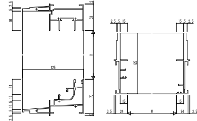
(9) 引違い窓 セフトバック枠 アンクルなし
