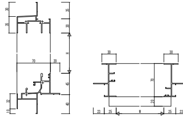
(7) 引違い窓・片引き窓・両軸片引き窓・引分け窓・自由片引き窓 鉄骨枠 半外付
