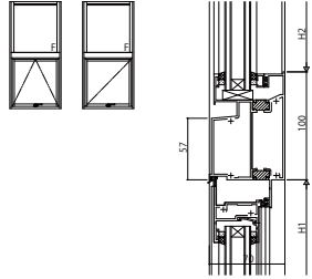
(15) FIX窓(内押縁)/ 突出し窓(ｶﾞﾗｯﾁ・ｸﾞﾚﾝ)・露出・隠ぺい)・すべり出し窓
