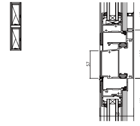
(23) たてすべり出し窓(ﾊﾞﾚｰﾀｰﾝﾄﾞﾙ・ｽﾘｯﾄ換気窓) /たてすべり出し窓(ﾊﾞﾚｰﾀｰﾝﾄﾞﾙ・ｽﾘｯﾄ換気窓)
