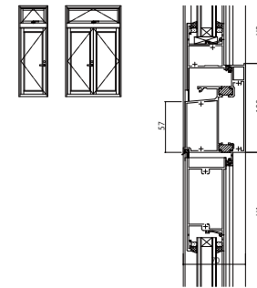
(27) 突出し窓/片開き・両開きドア(一般・防音)
