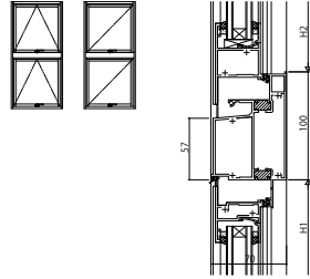
(16) 突出し窓(ｶﾞﾗｯﾁ・露出)・すべり出し窓/ 突出し窓(ｶﾞﾗｯﾁ・露出)・すべり出し窓
