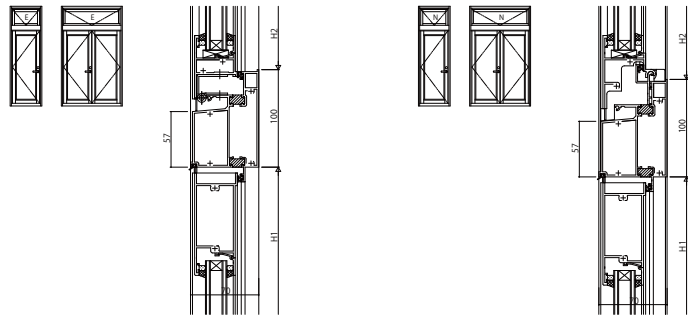
(25) 外倒し窓(露出・隠ぺい)/片開き・両開きドア(一般・防音) (26) 内倒し窓(一般・露出)/片開き・両開きドア(一般・防音)
