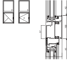
(17) FIX窓(内押縁)/外開き窓・たてすべり出し窓
