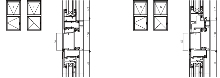
(18) 外倒し窓(一般・露出・隠ぺい)/外開き窓・たてすべり出し窓 (19) 内倒し窓(一般・露出)/外開き窓・たてすべり出し窓
