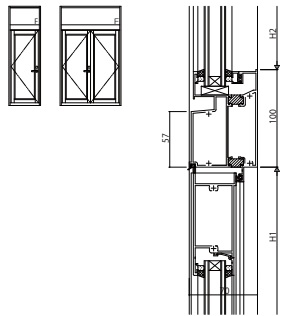
(24) FIX窓(内押縁)/片開き・両開きドア(一般・防音)
