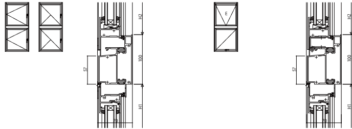
(21) 外開き窓・たてすべり出し窓/外開き窓・たてすべり出し窓 (22) 外倒し窓(露出・隠ぺい)/すべり出し窓(ｶﾞﾗｯﾁ・ｸﾞﾚﾝ)
