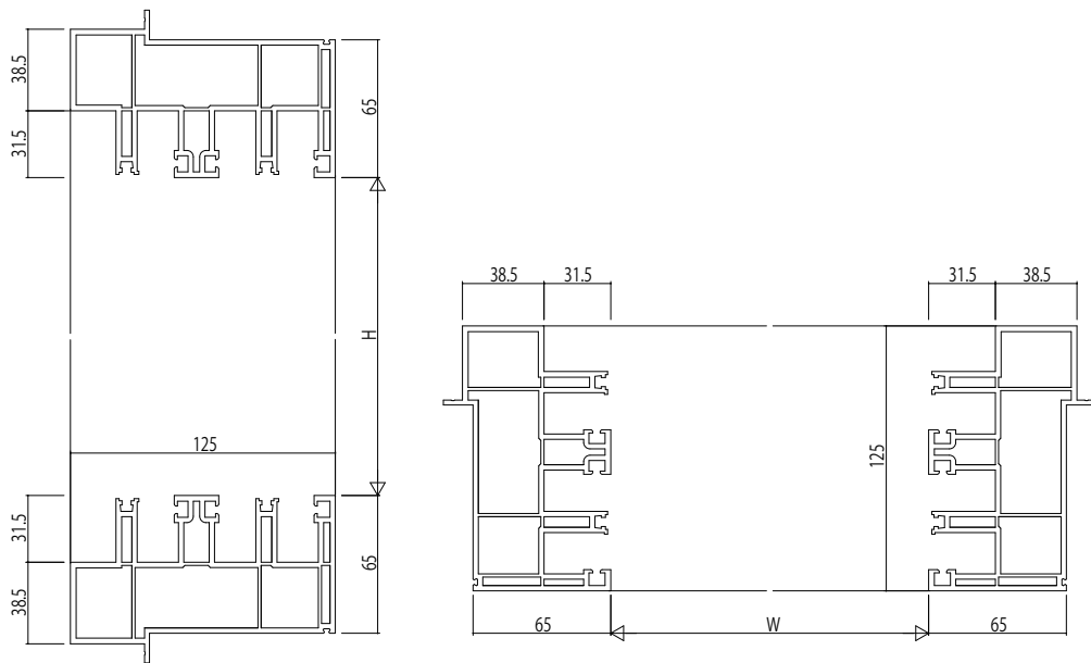
(1) 引違い・片引き(内動)・両袖片引き(内動) つらいち枠 アングルなし
