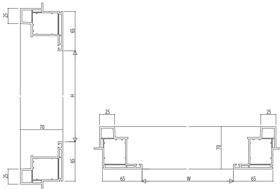
(3) 外倒し・たてすべり出し・外開き・片開きドア(かまち) つらいち枠 アングルなし
