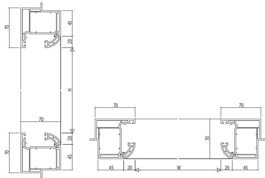
(2) FIX つらいち枠 アングルなし
