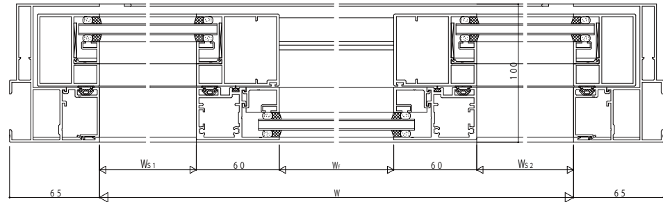
煙返し無
