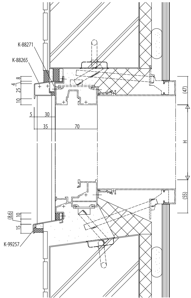
見切縁 35・RC納まり
