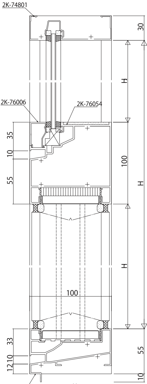
2K-76052 下枠 FIX窓／ガラスブロック
