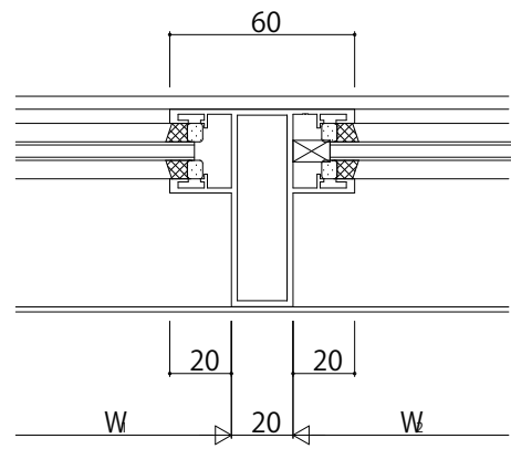
たて中骨
