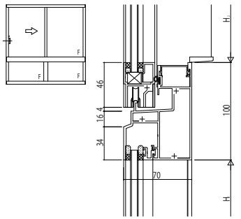
(9) 突出し【排煙窓・隠ぺい】/ F I X
