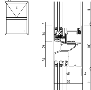
(13) 固定がらり【ルーバータイプ】/ F I X
