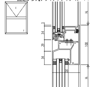
(12) 固定がらり【ブラインドタイプ】/ F I X
