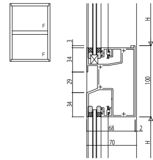
(10) すべり出し / F I X
