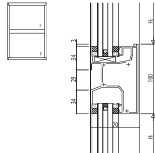
(11) たてすべり出し / F I X
