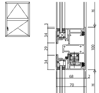
(17) 突出し【排煙窓・隠ぺい】/ たてすべり出し
