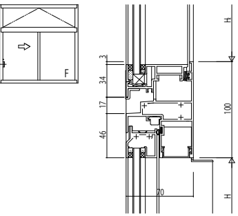
(7) 外倒し・突出し【排煙窓・隠ぺい】/ F I X 固定がらり【ブラインドタイプ・ルーバータイプ】/ F
