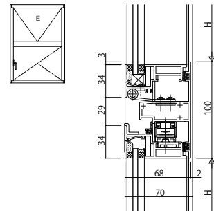
(16) 外倒し【排煙窓・隠ぺい】/ たてすべり出し
