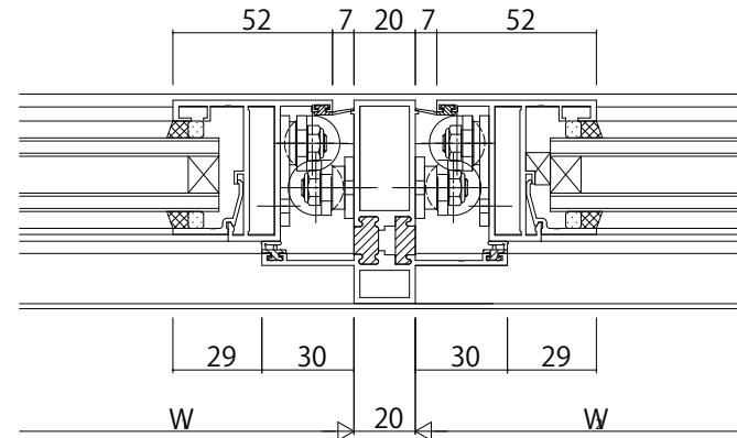
たて中骨
