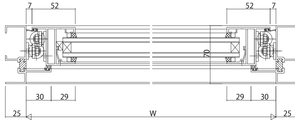
たて中骨
