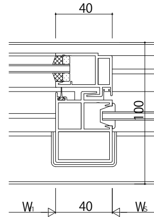
Bタイプ召合せかまち
