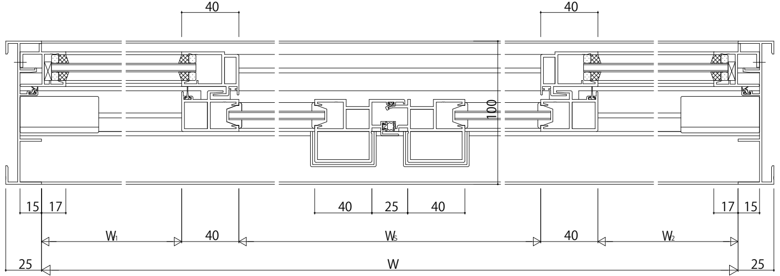
Aタイプ召合せかまち
