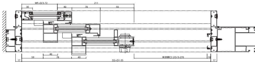
C-C 断面(開戸時)
