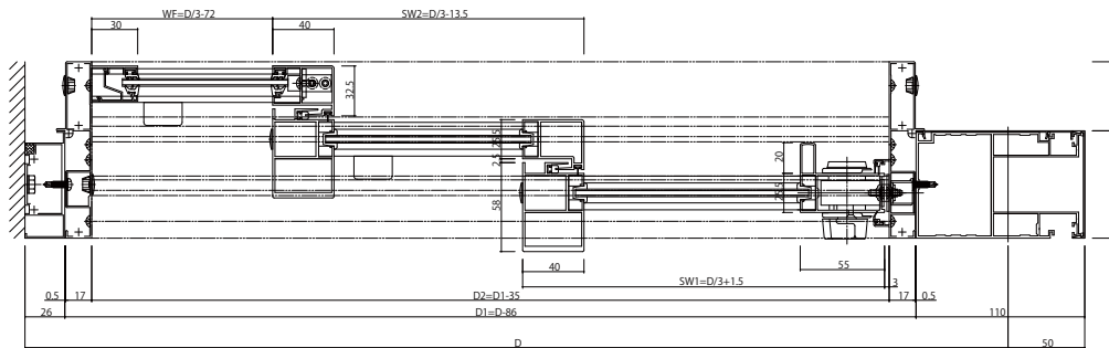
C-C 断面(閉戸時)
