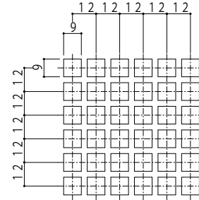
有効開口率55%以上 パンチング詳細
