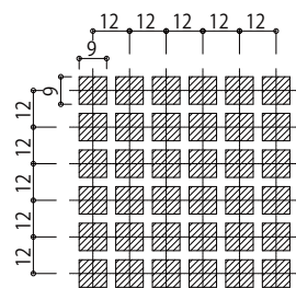
パンチング詳細
