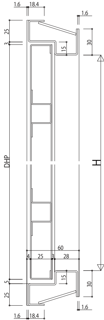
点検口側
