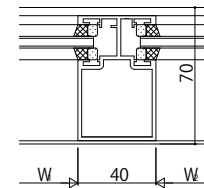
たて骨(40見付)
