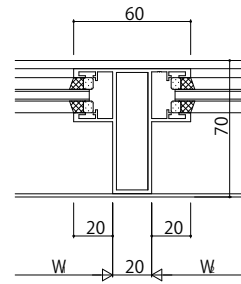
たて骨
