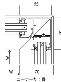
コーナーたて骨
