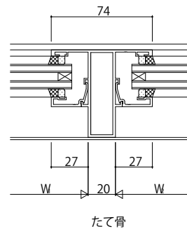
たて骨
