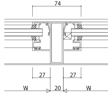
たて中骨
