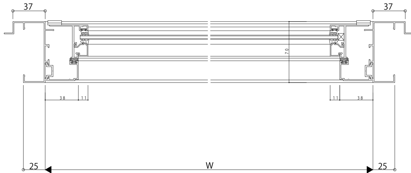
たて骨部(オーニング+FIX)
