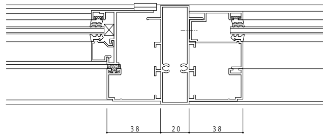
たて骨部(オーニング+FIX)
