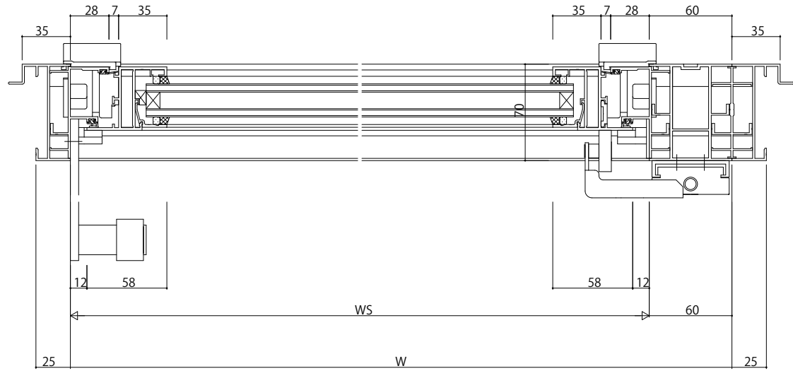
B-B断面
