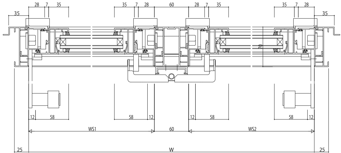
B-B断面
