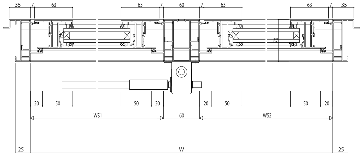
A-A断面
