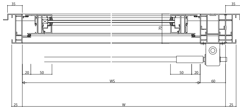
A-A断面
