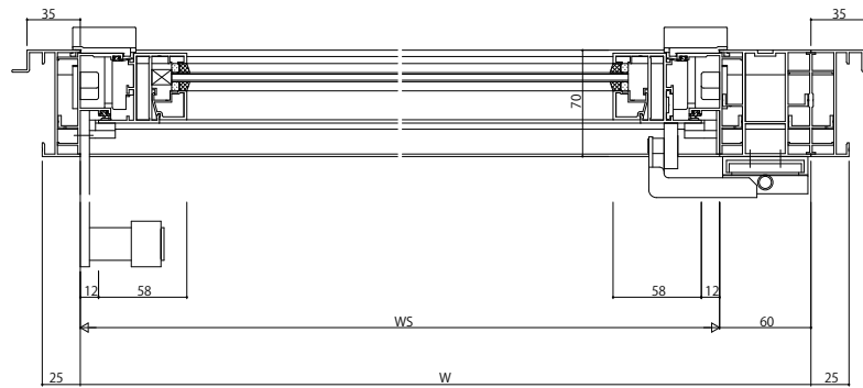
B-B断面
