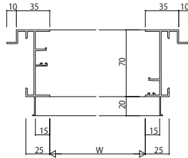
ALC 枠 アングル付 2枚建
