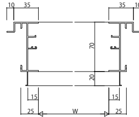
ALC 枠 アングル付 4枚建
