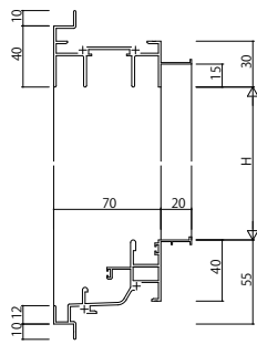
ALC 枠 アングル付
