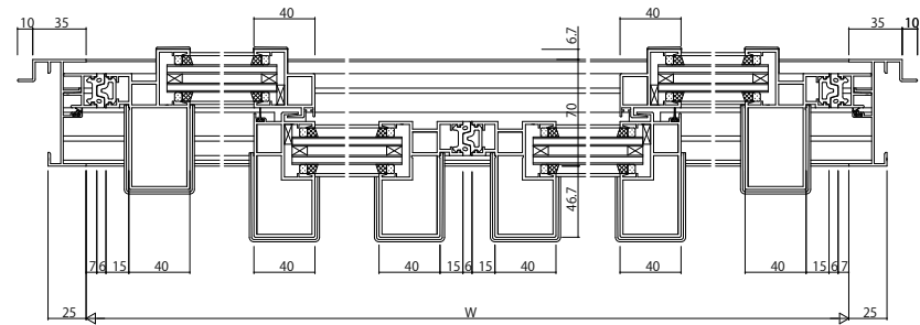
4枚建 Dタイプの場合
