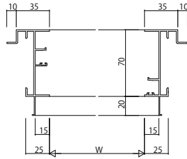
ALC 枠 アンクル付 2枚建
