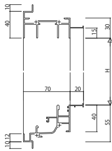
ALC 枠 アンクル付
