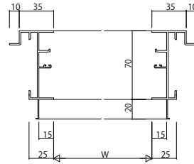
ALC 枠 アンクル付 4枚建
