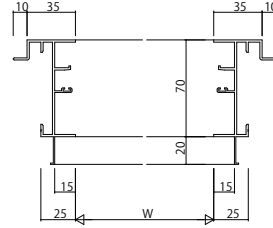
ALC 枠 アングル付 4枚建
