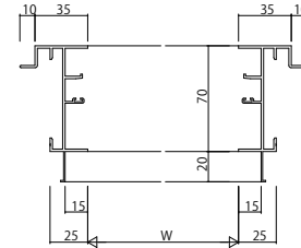
ALC 枠 アンクル付 4枚建
