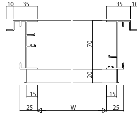
ALC 枠 アンクル付 2枚建
