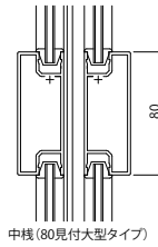
中棧 (80見付大型タイプ)
