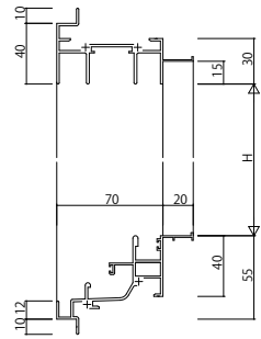
ALC 枠 アンゲル付
