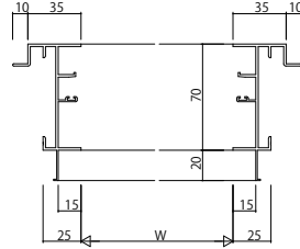
ALC 枠 アンゲル付 4枚建
