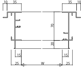
ALC 枠 アンゲル付 2枚建
