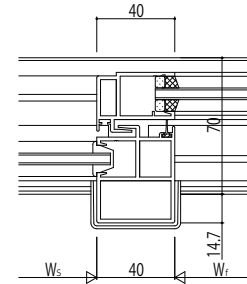
Bタイプ召合せかまち
