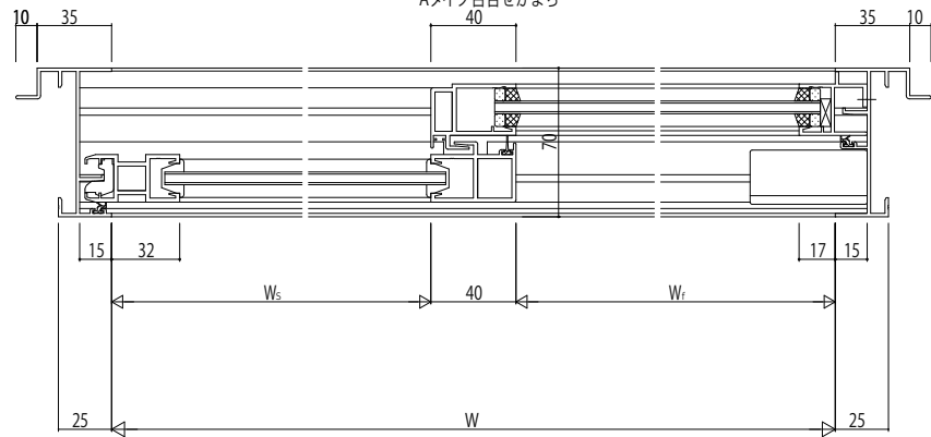
Aタイプ召合せかまち
