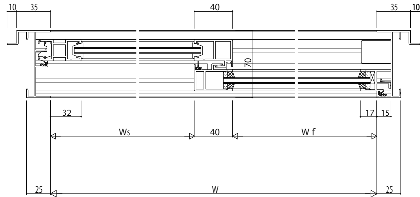
中棧 (80見付)
