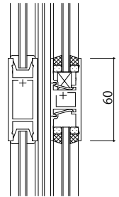
中棧 (60見付)
