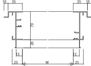
ALC枠 アンガル付 2枚建
