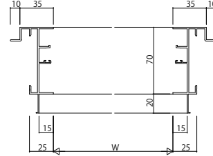
ALC枠 アンガル付 4枚建
