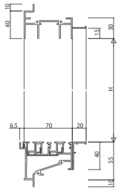
ALC枠 アンガル付
