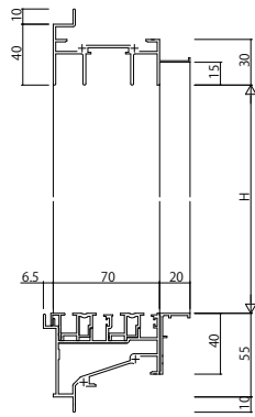
ALC枠 アンクル付
