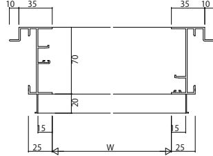
ALC枠 アングル付 2枚建
