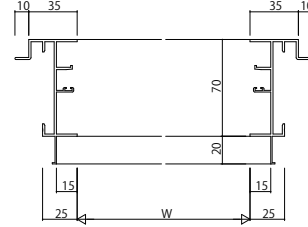
ALC枠 アンクル付 4枚建
