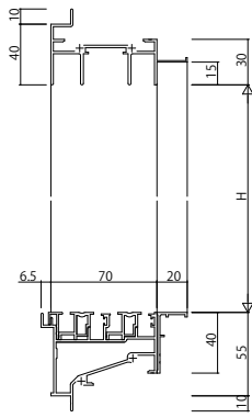
ALC枠 アンクル付
