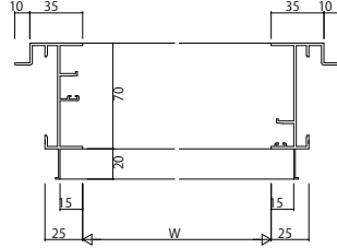
ALC枠 アンクル付 2枚建
