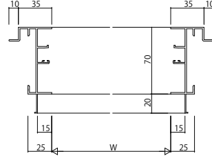
ALC枠 アンゲル付 4枚建
