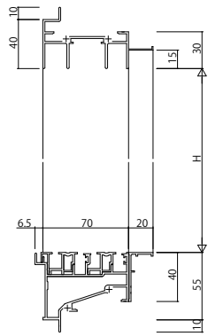
ALC枠 アンゲル付
