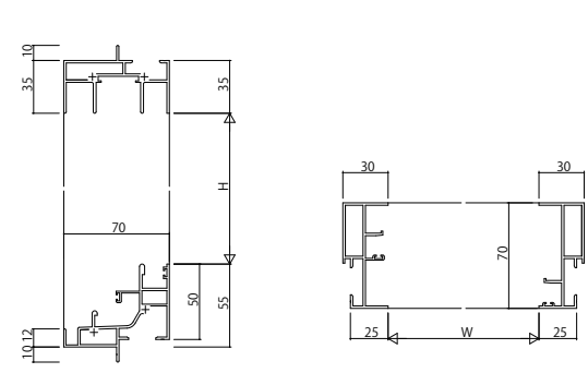
(5) 引違い窓・片引き窓 つらいち枠 アンガルなし
