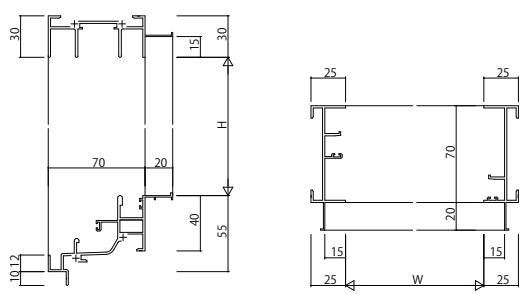
(1) 引違い窓・片引き窓 RC枠 アンガル付
