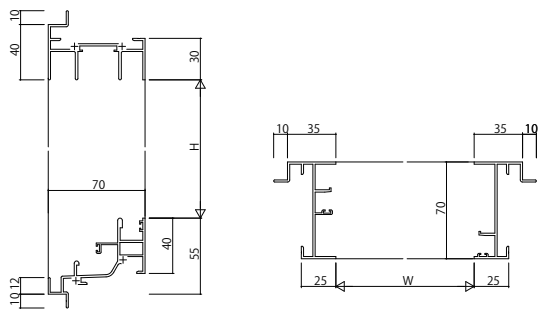
(4) 引違い窓・片引き窓 ALC枠 アンガルなし
