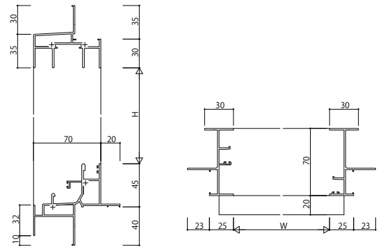
(7) 引違い窓 鉄骨半外付枠 アンガルなし
