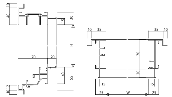
(3) 引違い窓・片引き窓 ALC枠 アンガル付
