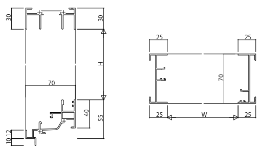
(2) 引違い窓・片引き窓 RC枠 アンガルなし
