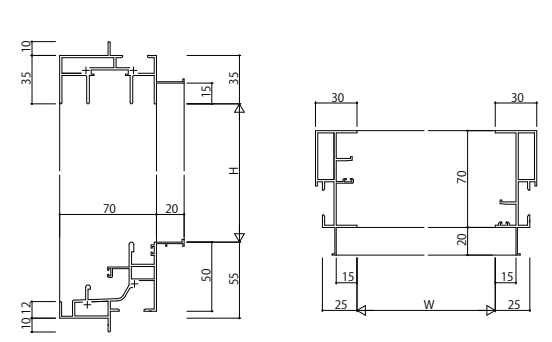
(6) 引違い窓 つらいち枠 アンガル付
