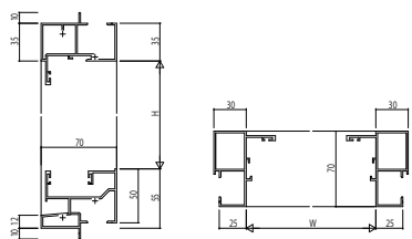
(5)FIX窓【内押鍵タイプ】 ついで枠 アングルなし
