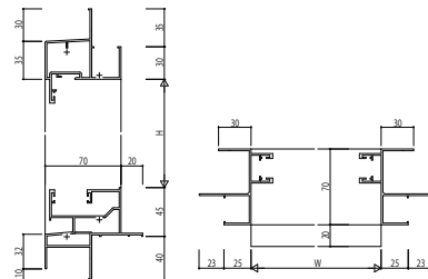
(6)FIX窓【内押鍵タイプ】 既設枠あり アングルなし
