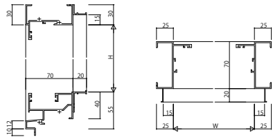
(1)FIX窓【内押鍵タイプ】 配格 アングル付
