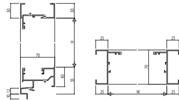
(2)FIX窓【内押鍵タイプ】 配格 アングルなし
