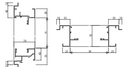
(8)FIX窓【外押鍵タイプ】 配格 アングルなし
