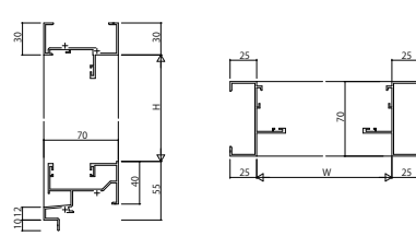
(7)FIX窓【外押鍵タイプ】 配格 アングルなし
