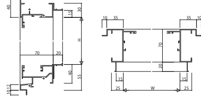
(3)FIX窓【内押鍵タイプ】 配格 アングル付
