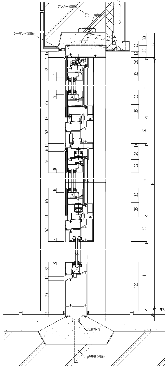
外倒し窓【排煙窓】/たてすべり出し窓FIX窓
