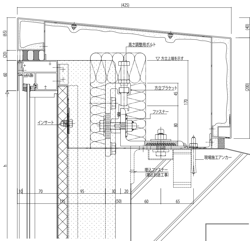
〈最上部 笠木納まり〉
