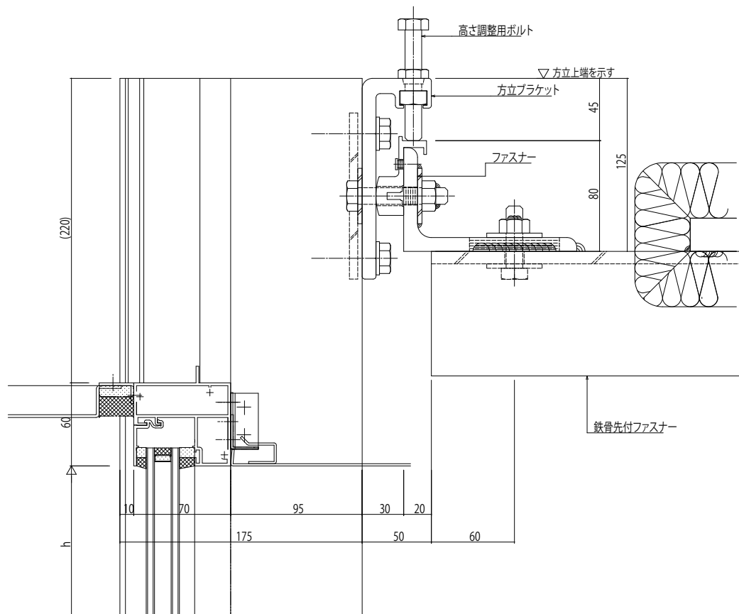
〈最上部 軒天納まり〉
