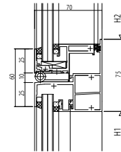
外倒し窓/FIX窓
