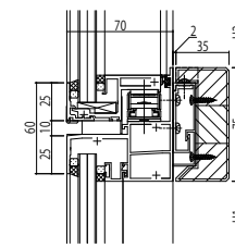
たてすべり出し窓/FIX窓
