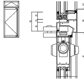
●突出し窓 (開べい) /ピボットヒンジドア
