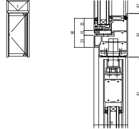
●外側し窓 (開べい) /フロアヒンジドア
