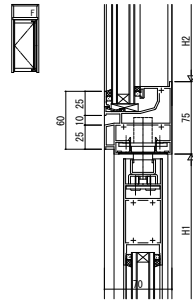
●FIX窓/自由開きドア【フロアヒンジドア】
