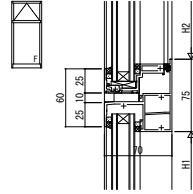
●突出し窓 (開べい) /FIX窓
