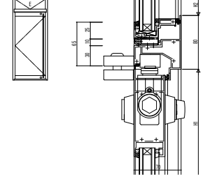
●外側し窓 (開べい) /ピボットヒンジドア
