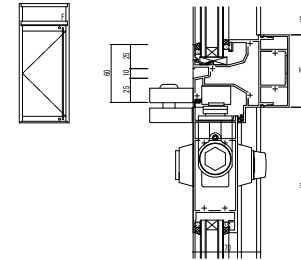
●FIX窓/ピボットヒンジドア 高強度難目仕様
