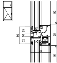
●FIX窓/たてすべり出し窓
