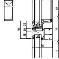
●外側し窓 (開べい) /FIX窓
