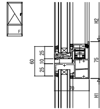
●たてすべり出し窓/FIX窓
