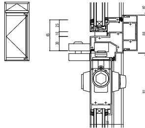
●突出し窓 (開べい) /ピボットヒンジドア 高強度難目仕様
