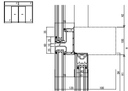
●FIX窓/自動ドア
