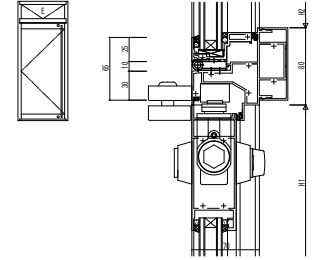
●外側し窓 (開べい) /ピボットヒンジドア 高強度難目仕様
