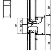
●FIX窓/FIX窓
