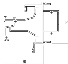
●FIX窓/ピボットヒンジドア高強度無目仕様
