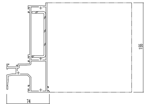
●FIX窓/自動ドア（上かまち隠べい）
