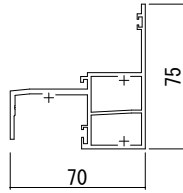
●可動窓/FIX窓
