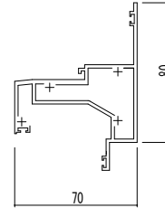
●外倒し窓・突出し窓（隠べい）/ピボットヒンジドア
