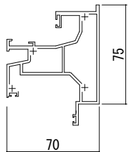
●FIX窓/片開きドア/両開きドア【かまちタイプ】
