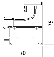
●FIX窓/自由開きドア【フロアヒンジドア】
