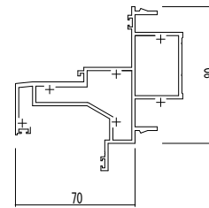
●外倒し窓・突出し窓（隠べい）/ピボットヒンジドア高強度無目仕様
