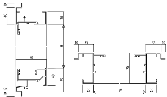
(4) FIX窓【内押縁タイプ】 ALC枠 アンガルなし
