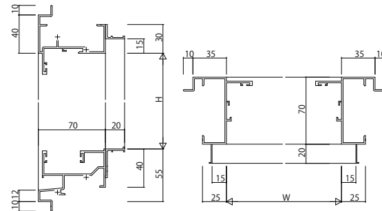
(3) FIX窓【内押縁タイプ】 ALC枠 アンガル付
