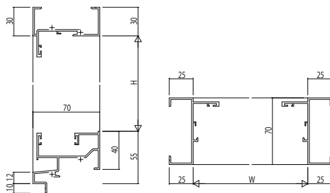
(2) FIX窓【内押縁タイプ】 RC枠 アンガルなし
