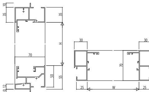
(5) FIX窓【内押縁タイプ】 つらもち枠 アンガルなし
