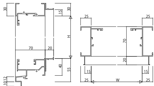
(1) FIX窓【内押縁タイプ】 RC枠 アンガル付
