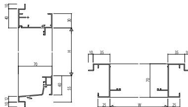
(30) ドア【ゆまぢタイプ】 ALC枠 アンガルなし
