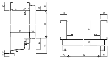
(30) ドア【ゆまぢタイプ】 ALC枠 アンガルなし
