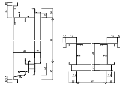
(21) 内側窓 ※2 ALC枠 アンガル付
