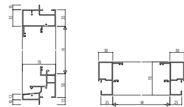
(23) 内側窓 ※2 つらいち枠 アンガルなし
