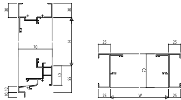
(27) ドア【ゆまぢタイプ】 RC枠 アンガル付
