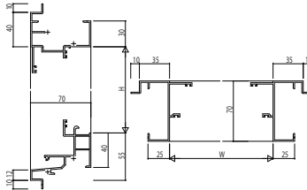
(25) 内側窓【排煙窓・隠ぺいオペレーター仕様】 ALC枠 アンガルなし
