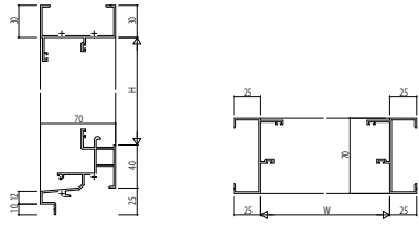
(24) 内側窓【排煙窓・隠ぺいオペレーター仕様】 RC枠 アンガルなし
