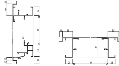
(26) 内側窓【排煙窓・隠ぺいオペレーター仕様】 つらいち枠 アンガルなし
