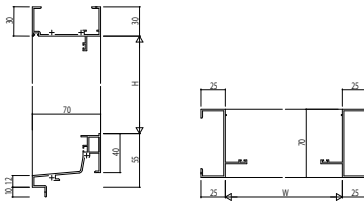
(31) ドア【ゆまぢタイプ】 つらいち枠 アンガルなし
