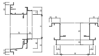
(29) ドア【ゆまぢタイプ】 ALC枠 アンガル付
