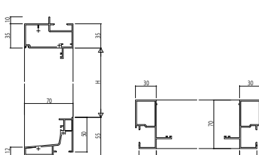
(31) ドア【ゆまぢタイプ】 つらいち枠 アンガルなし
