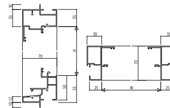
(26) 内側窓【排煙窓・隠ぺいオペレーター仕様】 つらいち枠 アンガルなし
