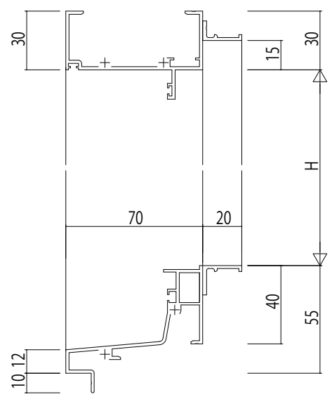
RC枠 アングル付
