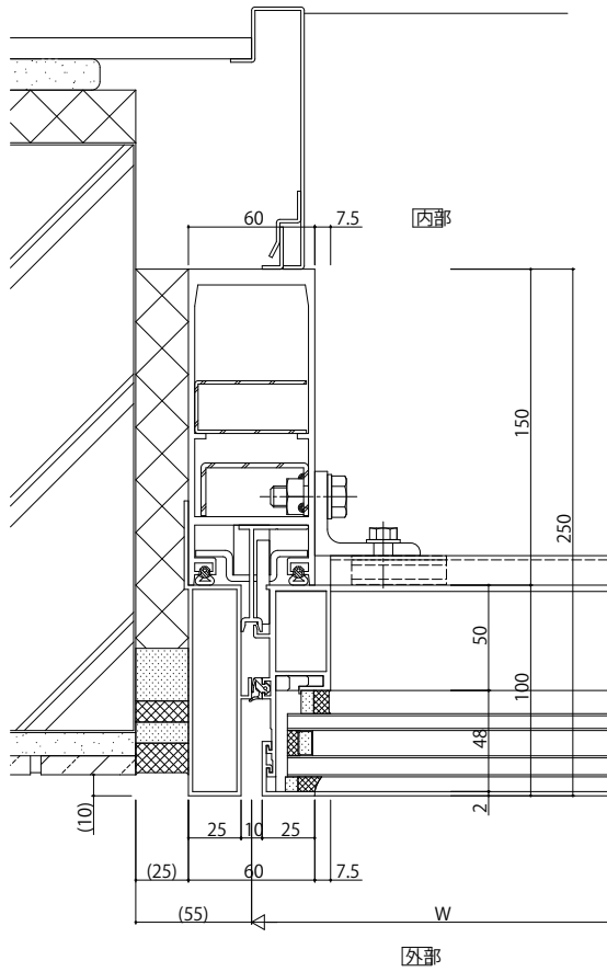
端部納まり
