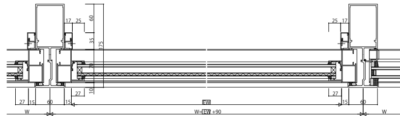
●FIX窓【内押縁タイプ】下段
