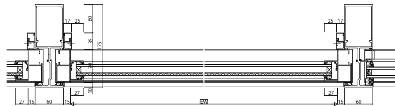
●FIX窓【内押縁タイプ】上段
