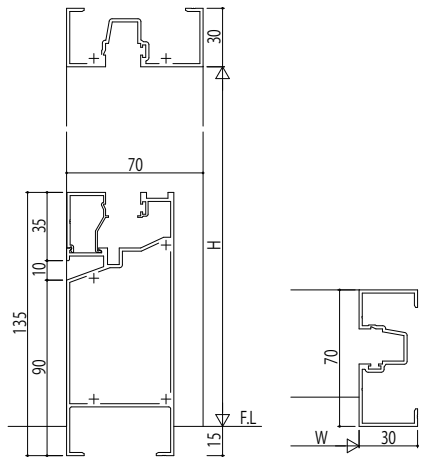
(5)FIX窓 幅木タイプ:135mm見付 RC枠アングルなし
