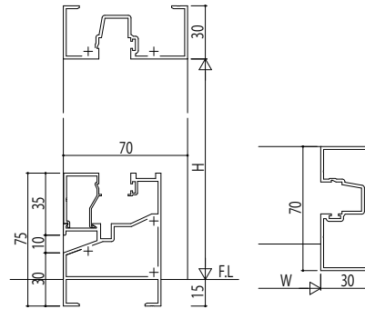
(3)FIX窓 幅木タイプ:75mm見付 RC枠アングルなし
