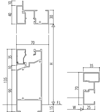
(6)FIX窓 幅木タイプ:135mm見付 ALC枠アングルなし
