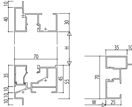
(2)FIX窓 下枠タイプ ALC枠アングルなし
