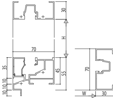
(1)FIX窓 下枠タイプ RC枠アングルなし
