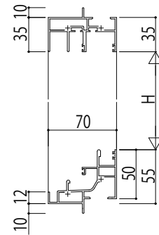
(5) 引違い窓 つらち 枠 アンゲルなし
