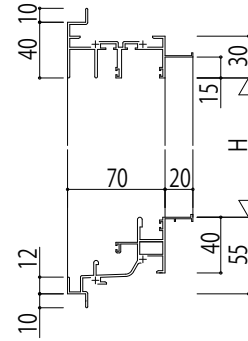
(3) 引違い窓 ALC 枠 アンゲル付
