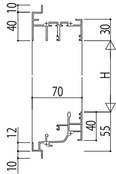
(4) 引違い窓 ALC 枠 アンゲルなし
