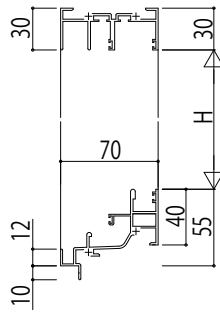
(2) 引違い窓 RC 枠 アンゲルなし
