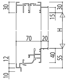
(1) 引違い窓 RC 枠 アンゲル付
